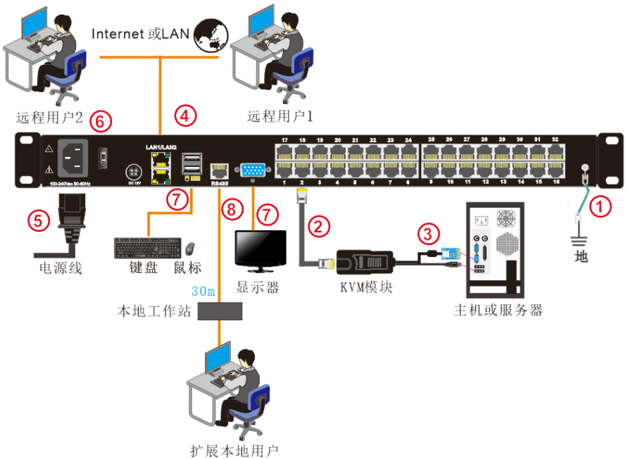
图 2.3 安装示意图
