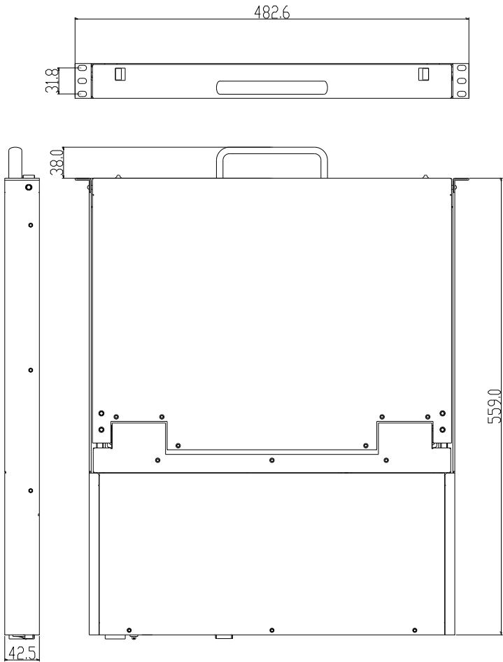
图 1-1.4 尺寸图
