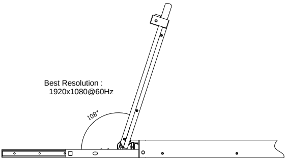
图 2-1.4 控制平台翻开角度
