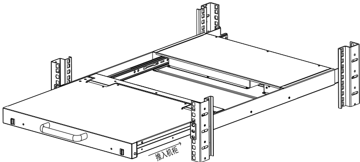
图 2-1.6 控制平台解锁示意图
