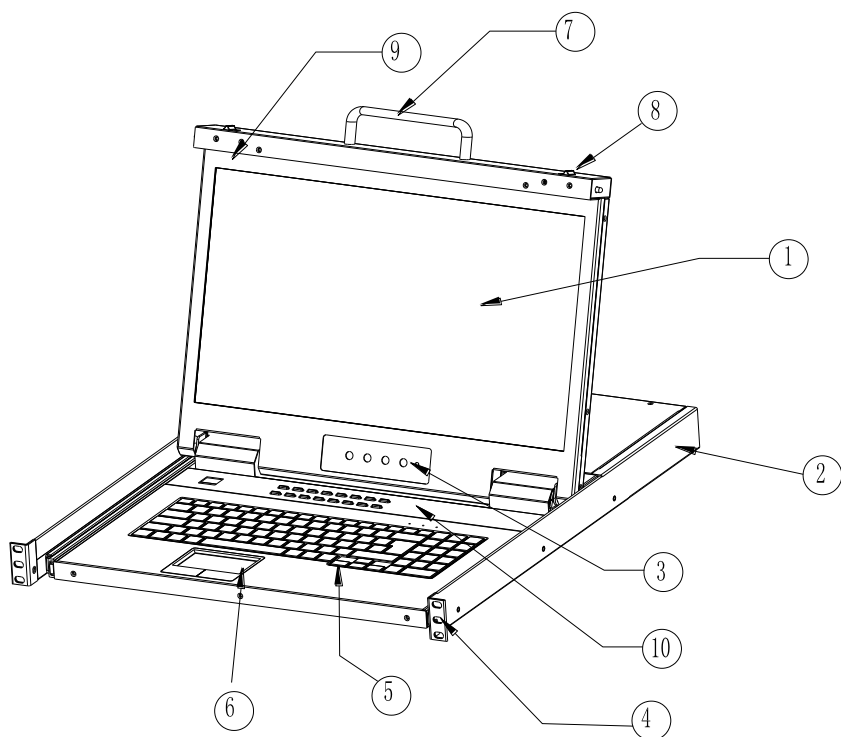
图 1-1 前视图
