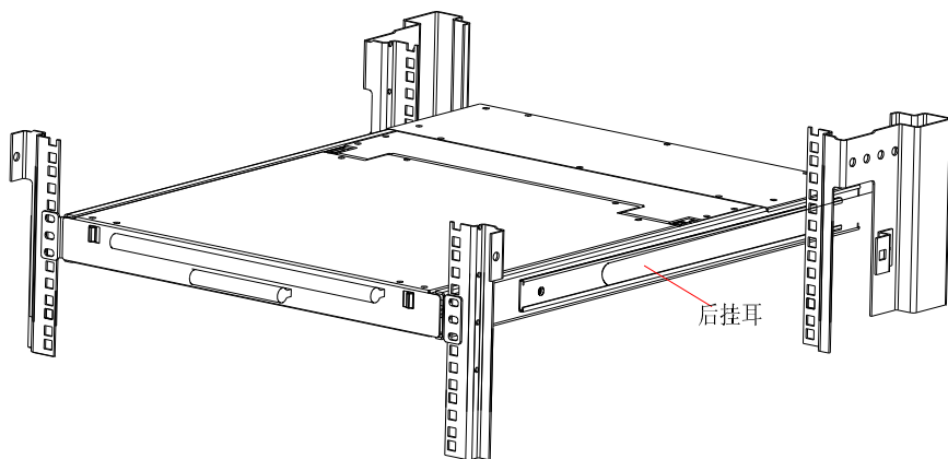
图 1-2.1 机架安装图(一)
