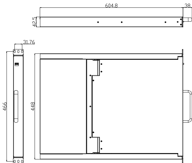
图 1-3 19"尺寸图
