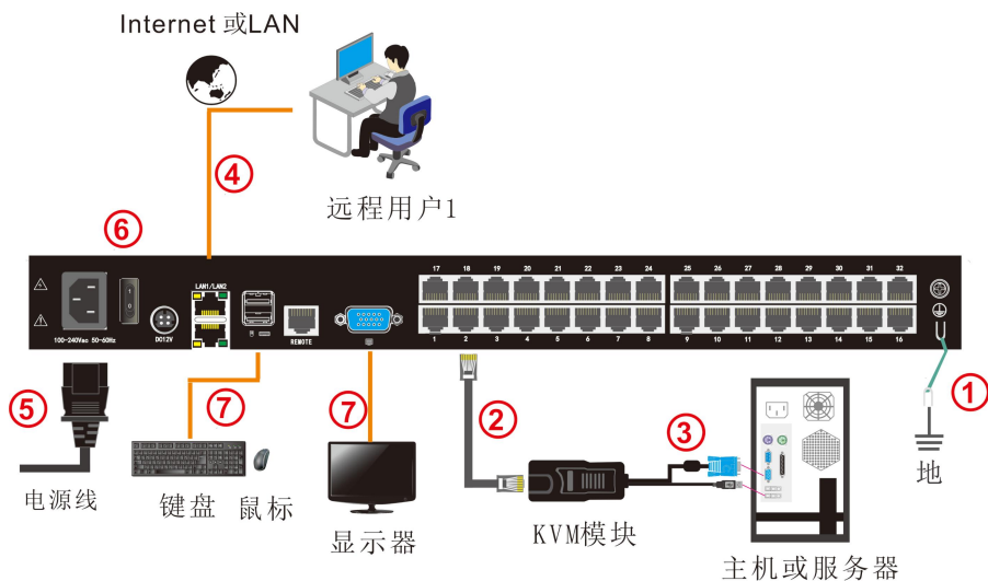
图 2-3 安装示意图
