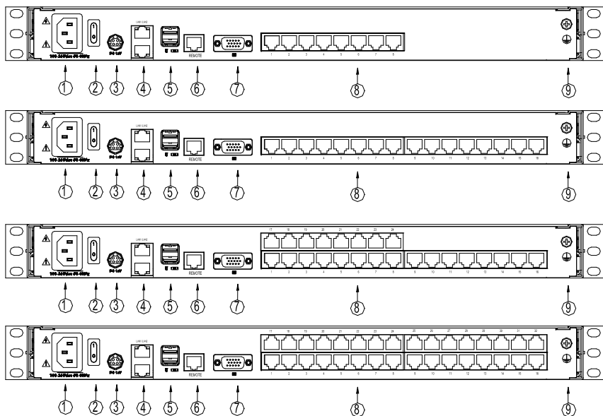
图 1-3 后视图
