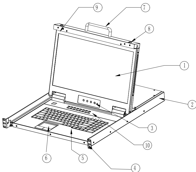
图 1-1 前视图
