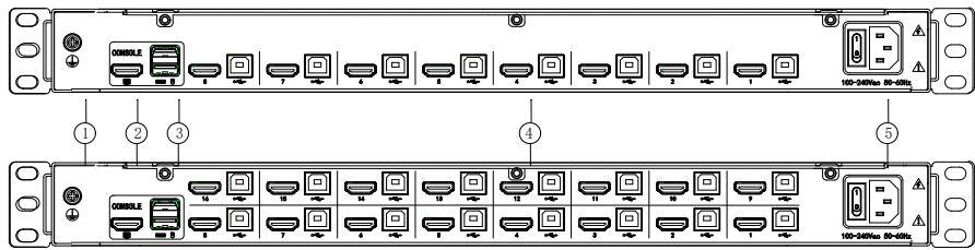
图 1-1.3 后视图
