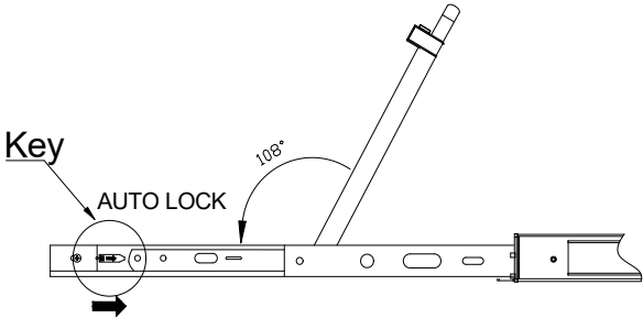
图 2-1.6 控制平台解锁示意图
