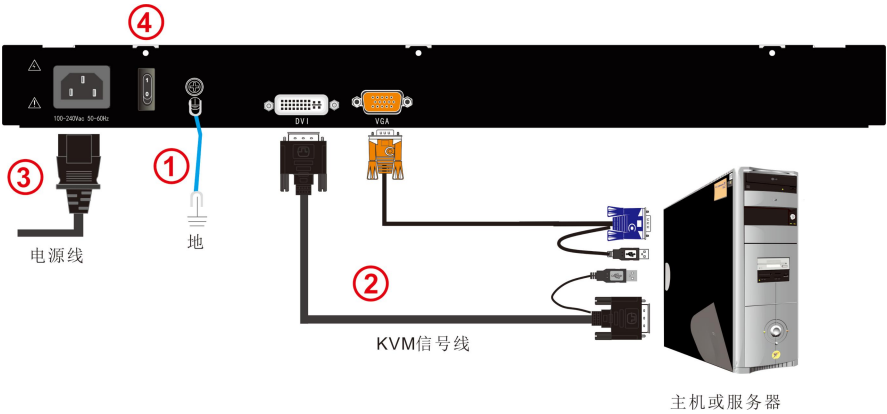
图 3-2 连线方式
