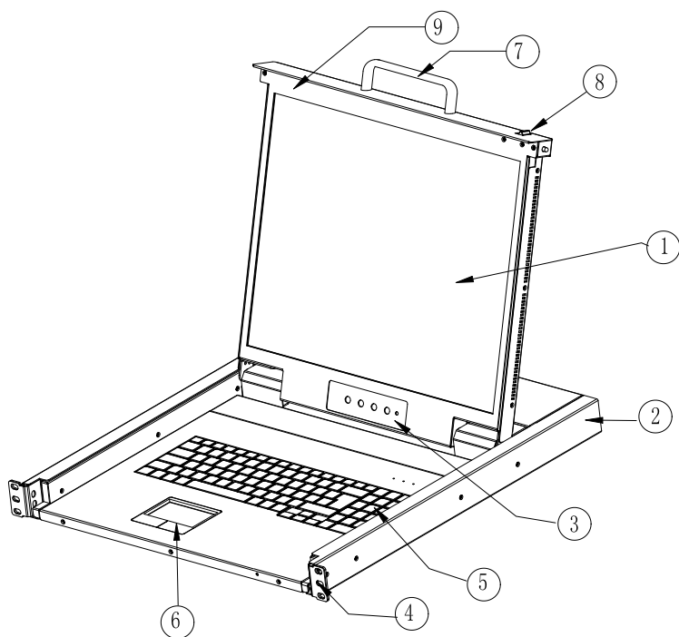
图 1-2 前视图
