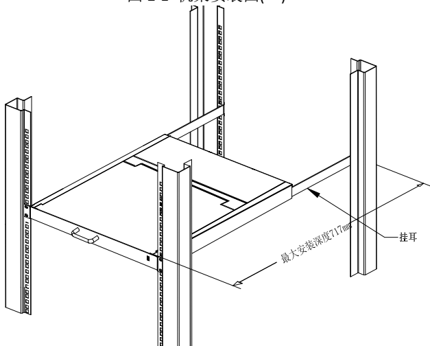
图 2-1 机架安装图(一)
