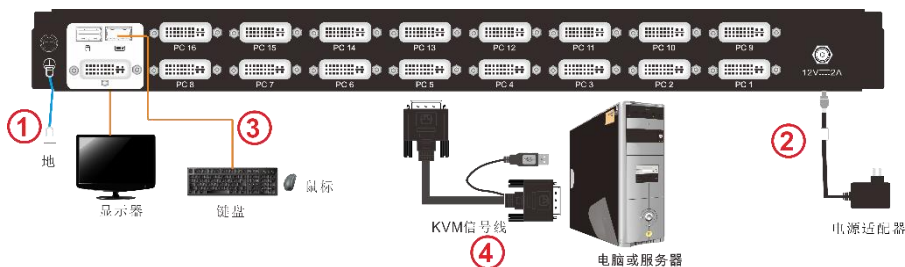
图 1.1 安装 KVM 配件图
