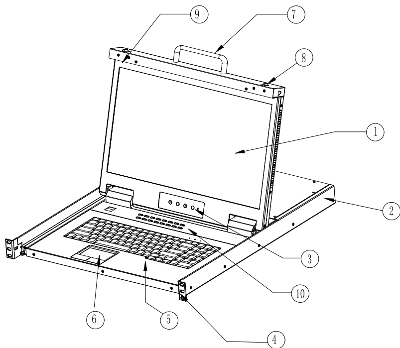
图 1-1.1 前视图
