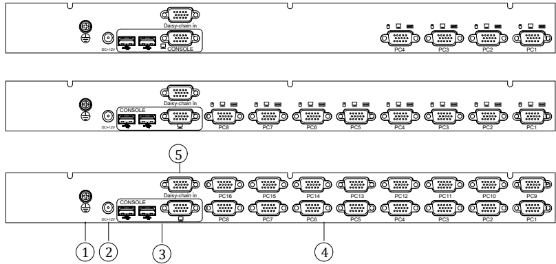
图 1-1.3 KVM 后视图
