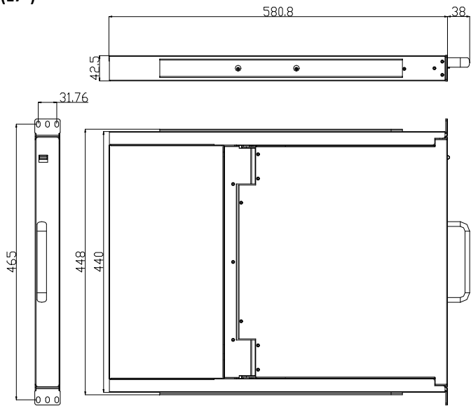
图 1-1.2 17"KVM 尺寸图
