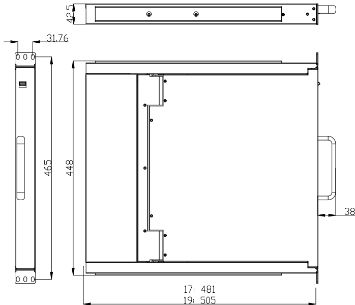
图 1-1 整体外观尺寸图
