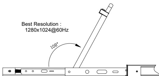
图 2-4 控制平台翻开角度
