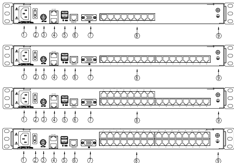
图 1-3 后视图
