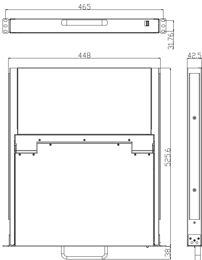
图 1-2 尺寸图
