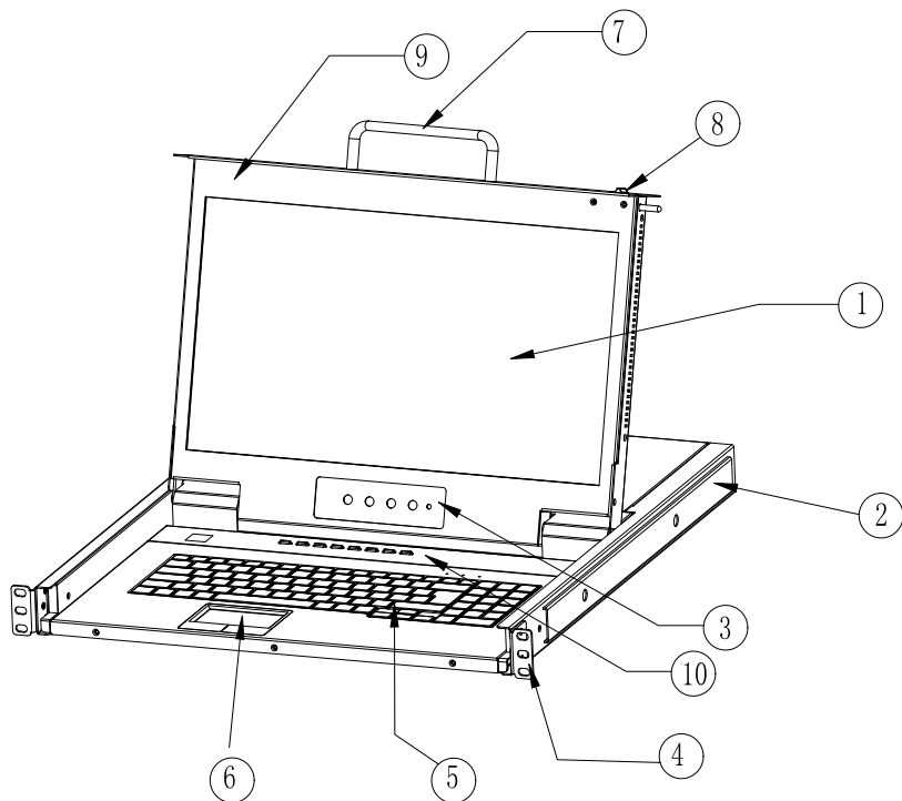
图 1-1 前视图
