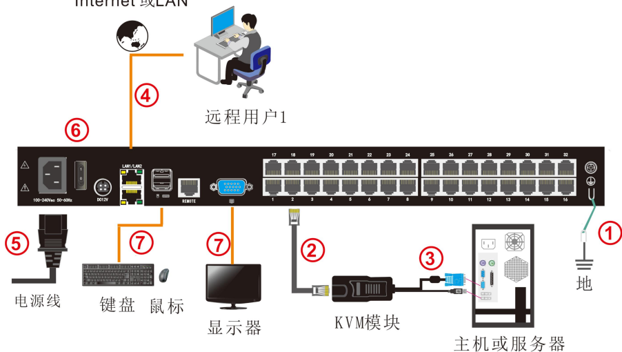
图 2-3 安装示意图
