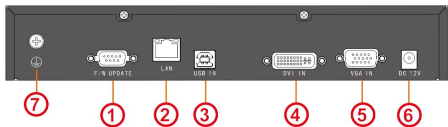
后视图
