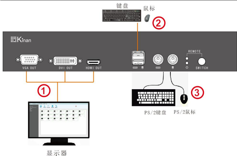
安装示意图
