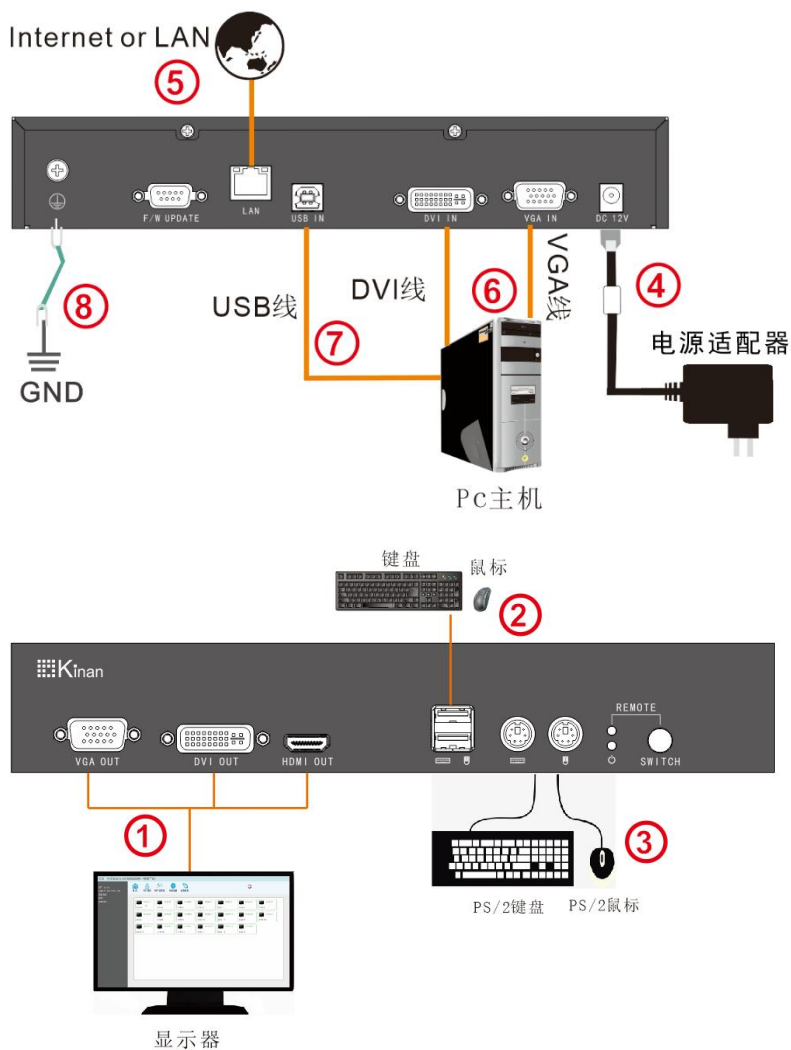
安装示意图
