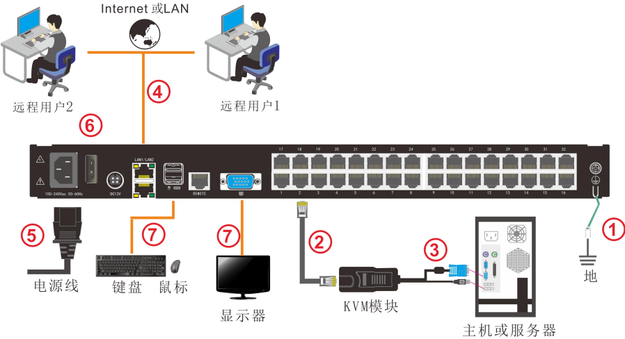
图 2-3 安装示意图
