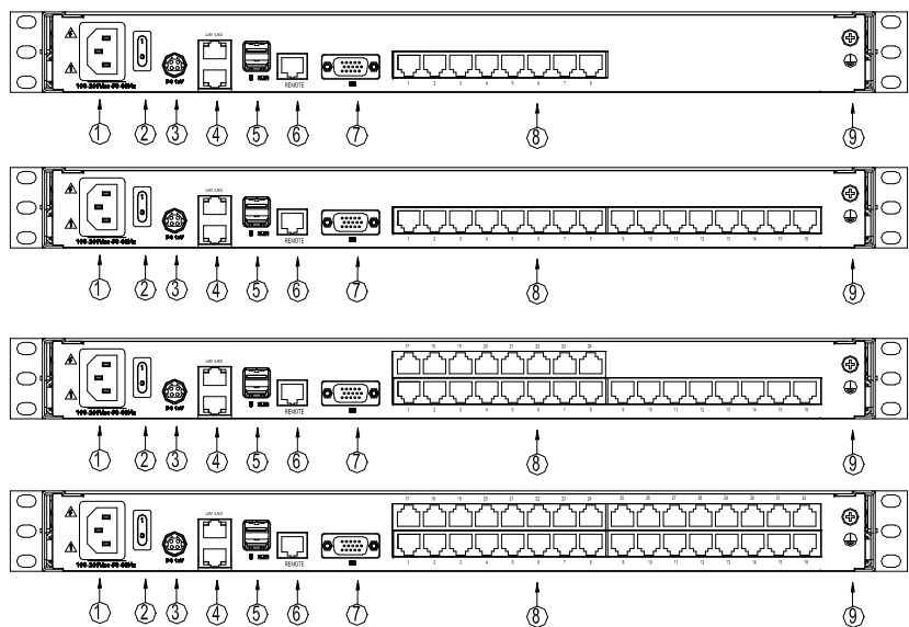
图 1-3 后视图
