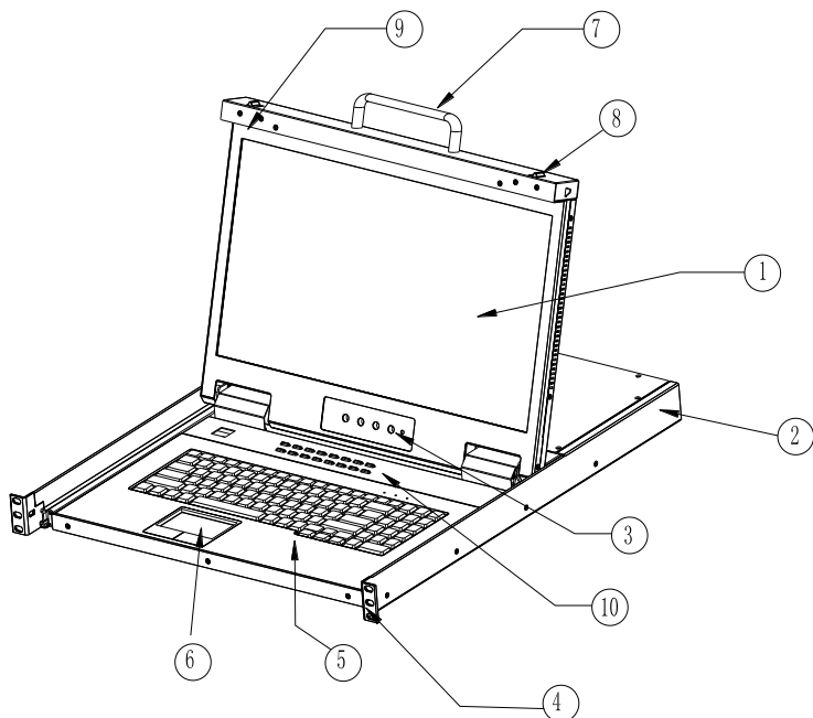
图 1-1.1 前视图
