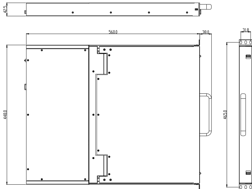
图 1-1.2 尺寸图
