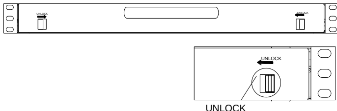
图 2-1.3 解锁方式
