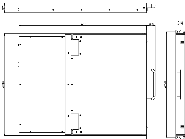
图 1-1 整体外观尺寸图
