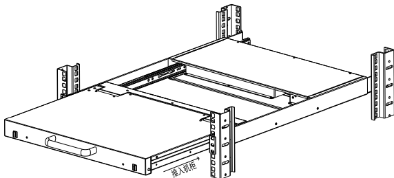
图 2-5 控制平台解锁示意图
