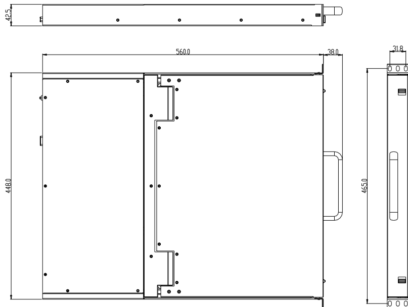
图 1-1.2 尺寸图
