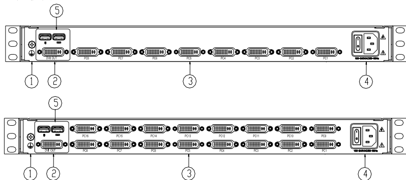
图 1-1.3 后视图
