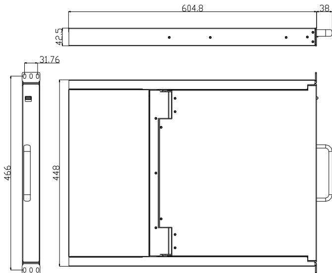
图 1-1.3 19"KVM 尺寸图
