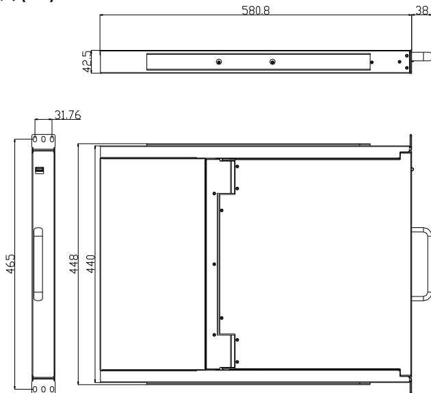
图 1-1.2 17"KVM 尺寸图
