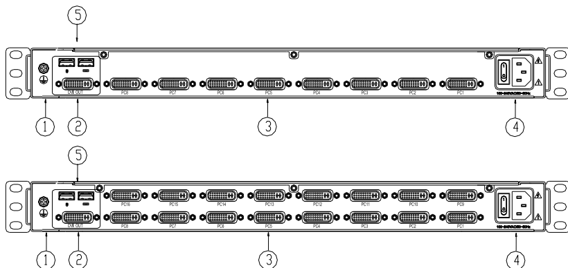
图 1-1.4 后视图
