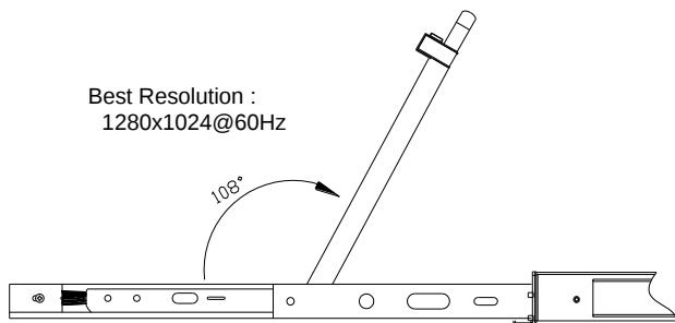
图 2-2.2 控制平台翻开角度
