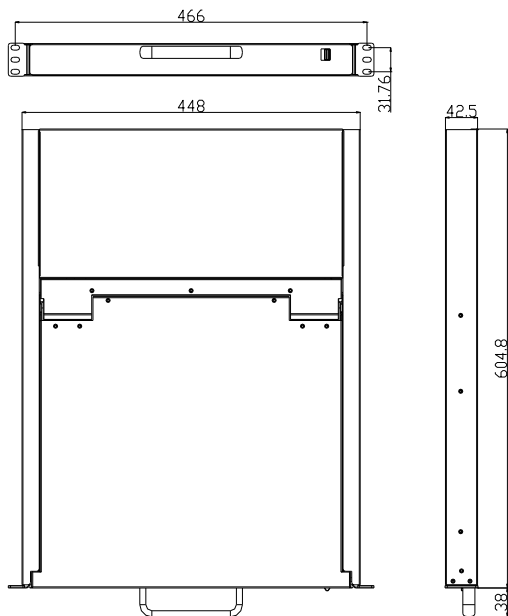
图 1-1.4 尺寸图
