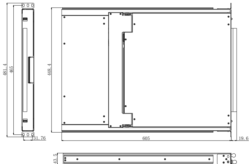
图 1-1.2 尺寸图
