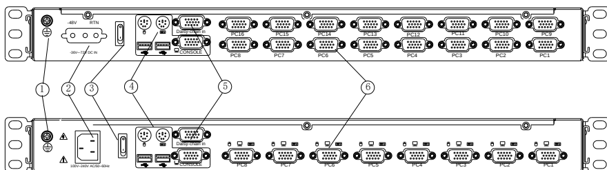
图 1-1.3 后视图
