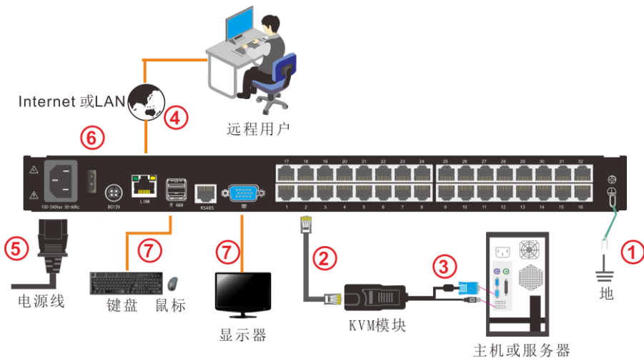
图 2-3 安装示意图
