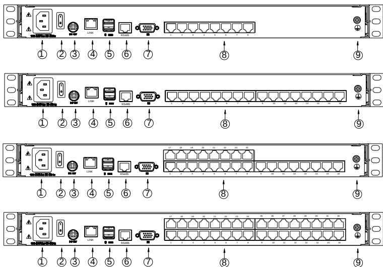
图 1-3 后视图
