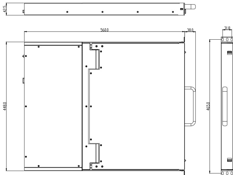
图 1-2 尺寸图
