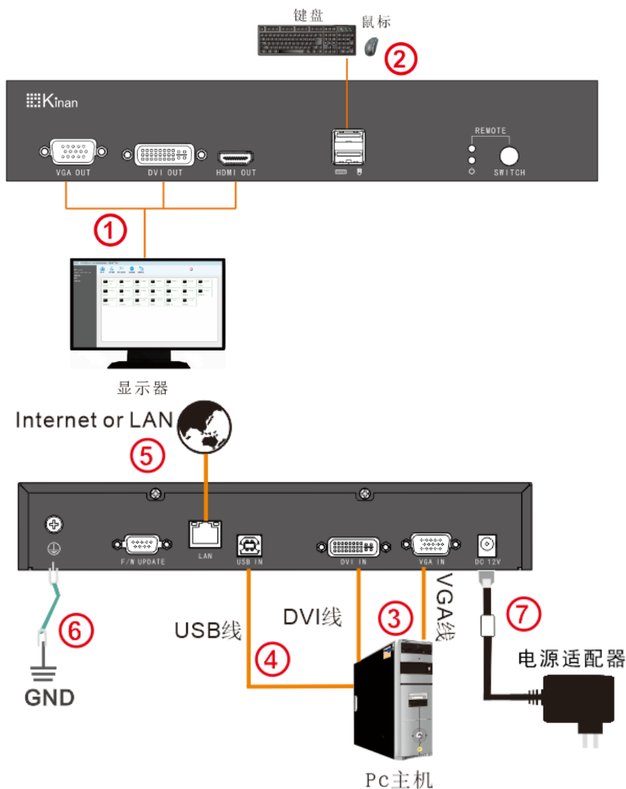
安装示意图
